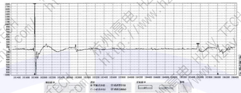
图 D.6 408.4m 局部放电脉冲波形
