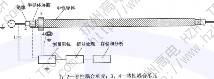
图 B.2 典型的局部放电测试系统
