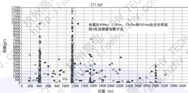
图 D.11 1.7U_0 局部放电点分布
