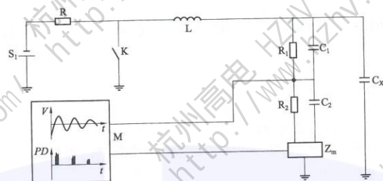
图1 直流激励式电缆振荡波局部放电测量系统组成示意图
