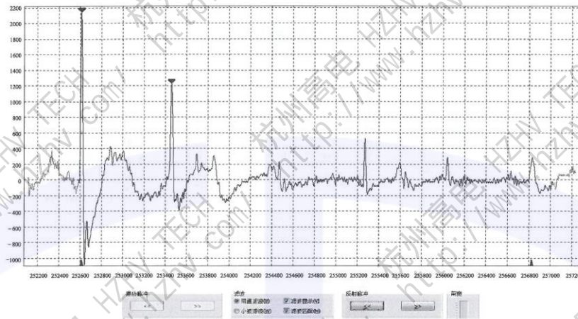
图 D.9 3014m 局部放电脉冲波形
