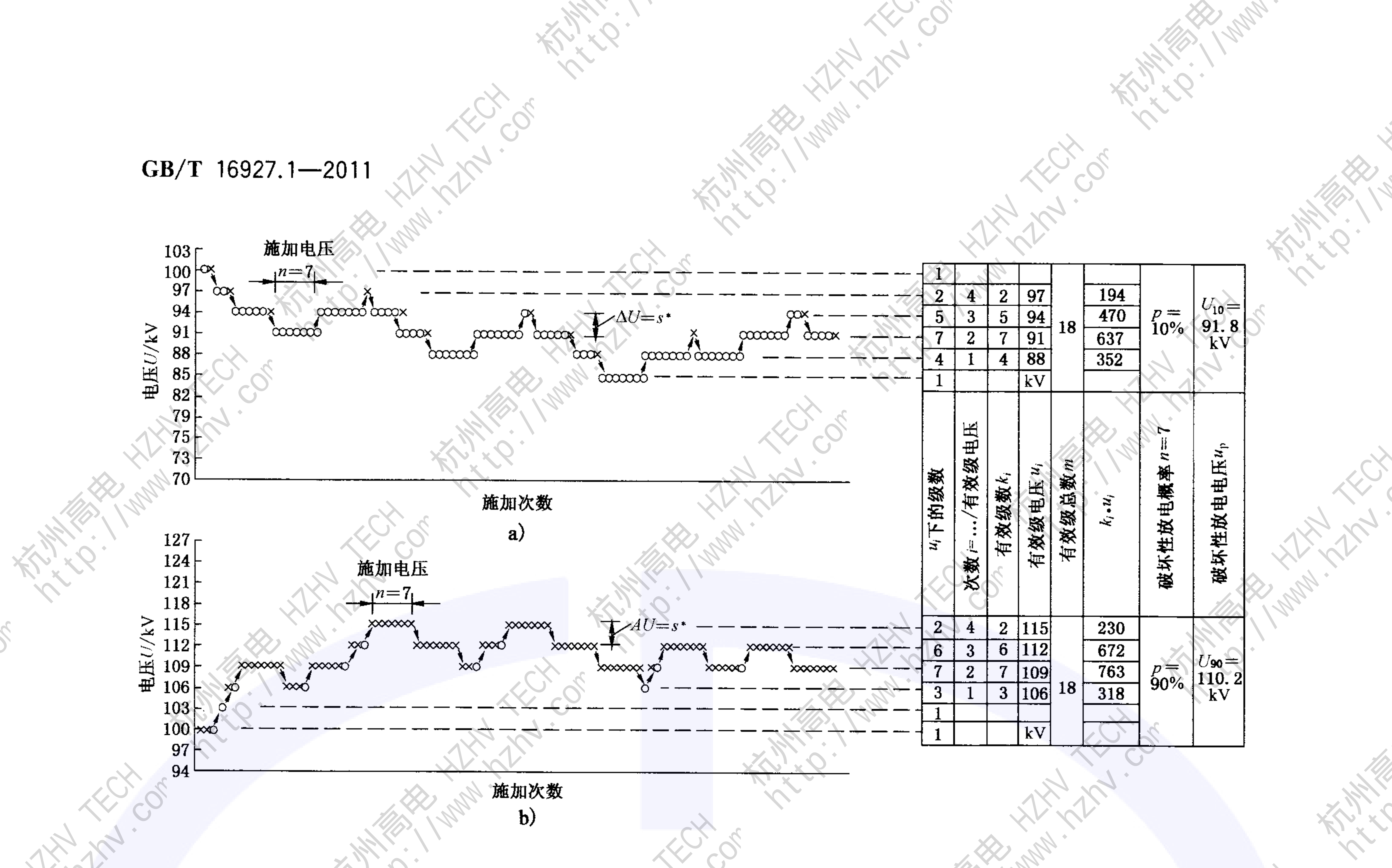
图 A.2 升降法试验分别确定 90%和 10%破坏性放电概率的示例(第二类试验)
