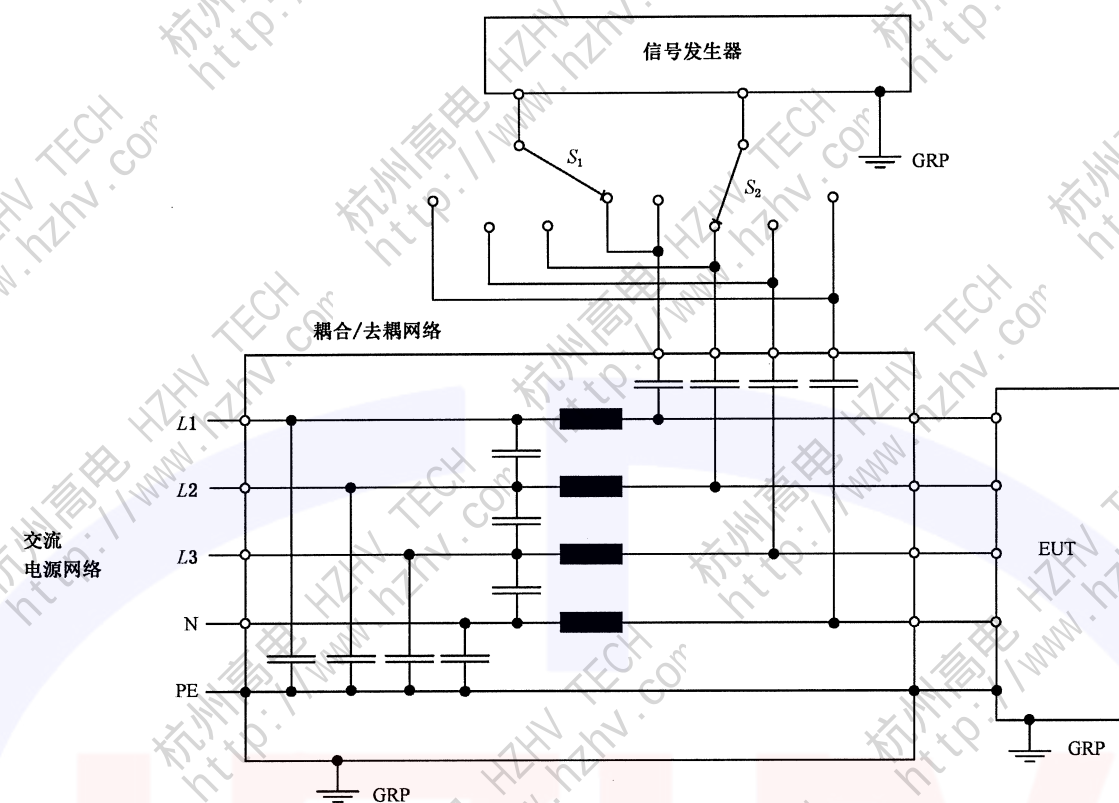
a) 使用接地参考平面的试验布置
