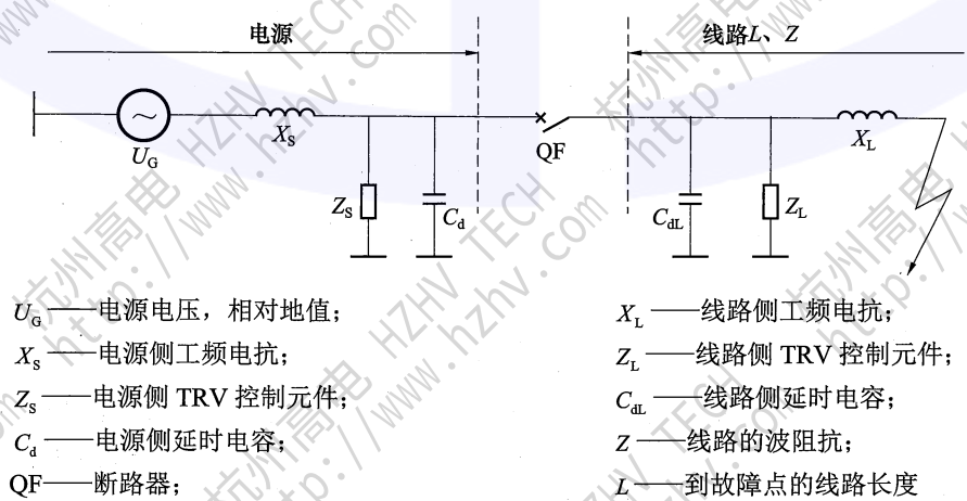
图 15 近区故障的基本回路
