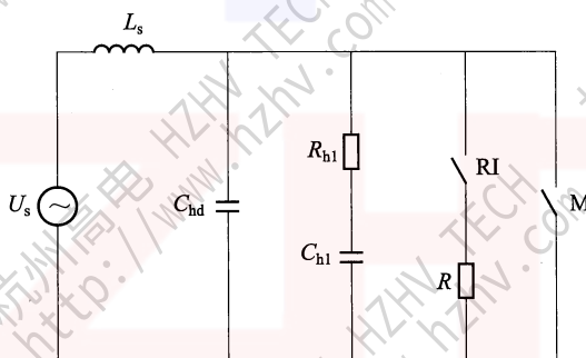
图 R.2 试验方式 T60 和 T100 的试验回路
