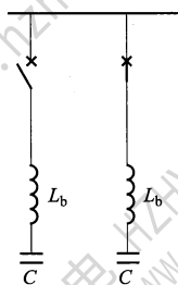
图 H.1 例 1 的回路图
