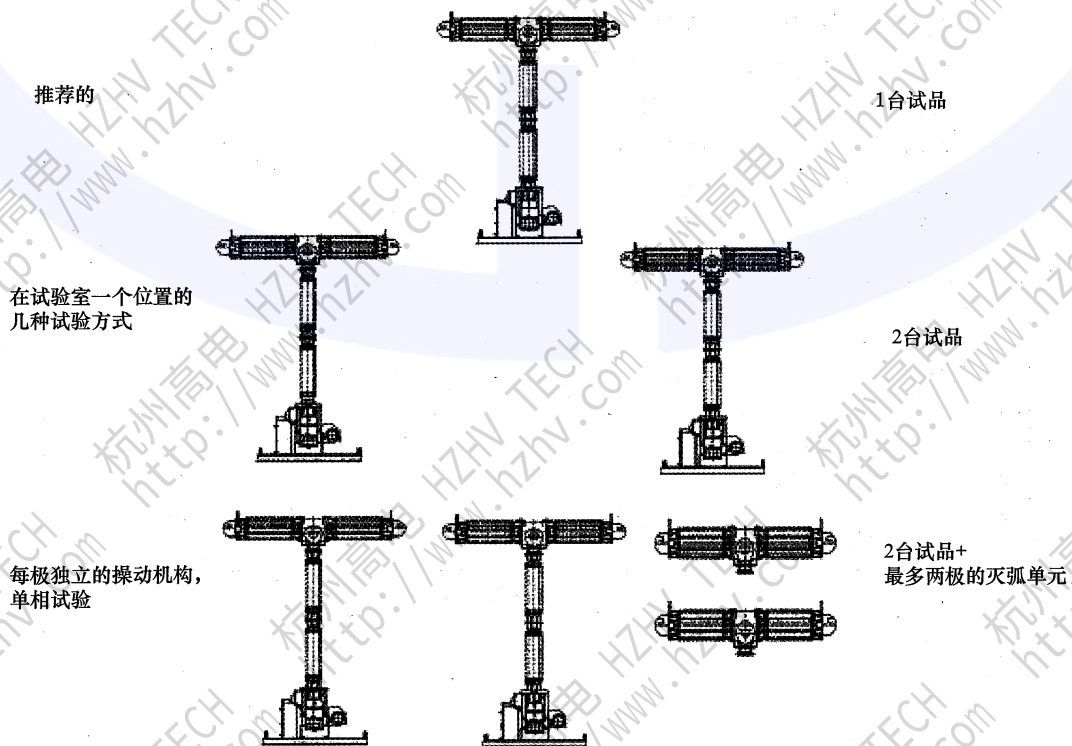
图 21 关合、开断和开合试验允许的试品数量（6.102 中规定的图示）
