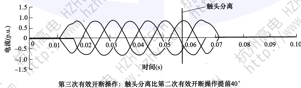
图 29 中性点非有效接地系统中（首开极系数 1.5）三相试验时三次有效对称开断操作的图形表示
