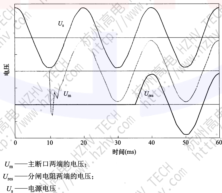
图 R.8 大短路电流开断操作的 TRV 波形
