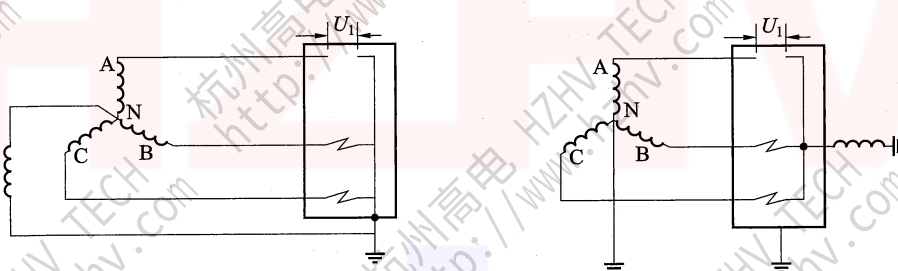
图 25 三相短路试验的试验回路的接地（首开极系数 1.5）
