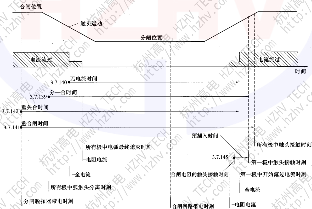
图 6 有开合电阻的断路器的合-分循环
