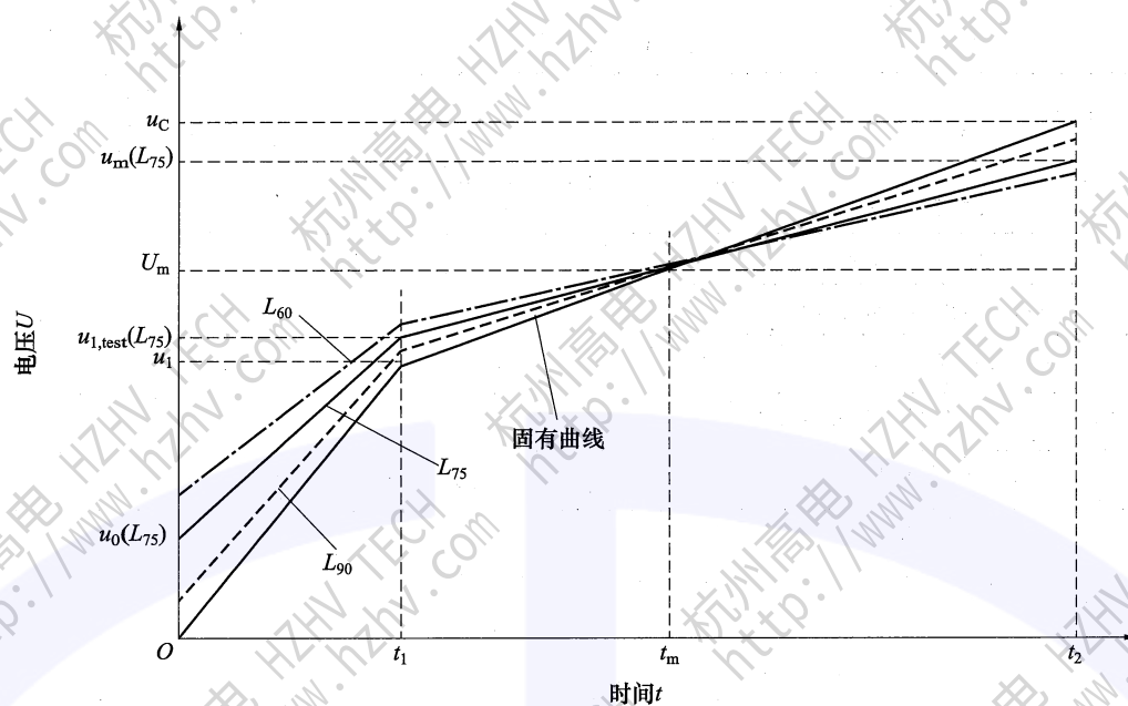
图 A.3 L_{90} 、 L_{75} 和 L_{60} 近区故障时电源侧 TRV 的实际曲线
