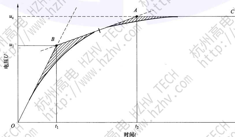
图 E.3 用四参数表示回路的预期瞬态恢复电压——E.2 的 c) 中 1) 的情况
