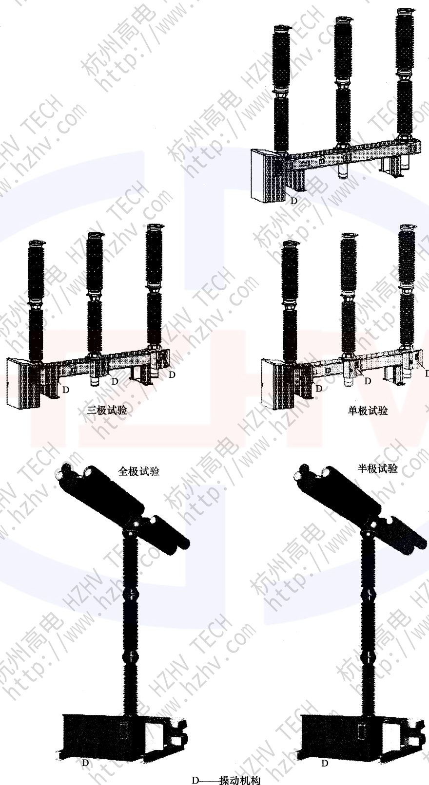
图 22 单个试品的定义 (见 DL/T 593—2016 的 3.2.1)
