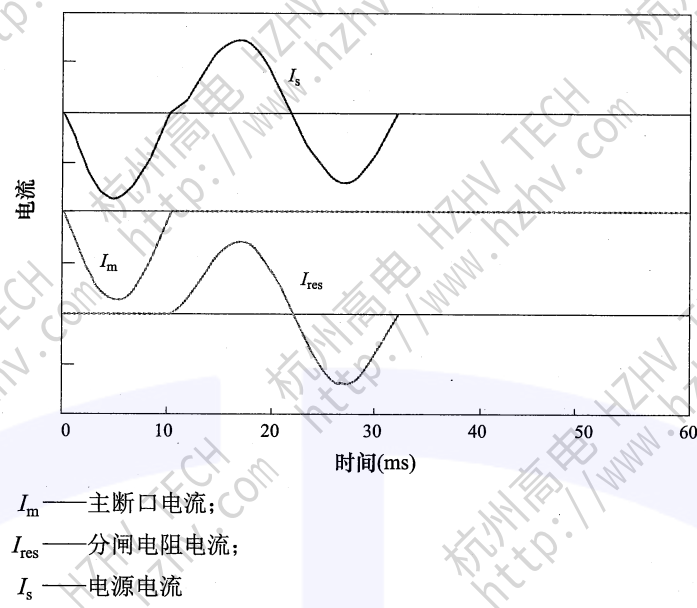
图 R.13 线路充电电流开断操作的电流波形
