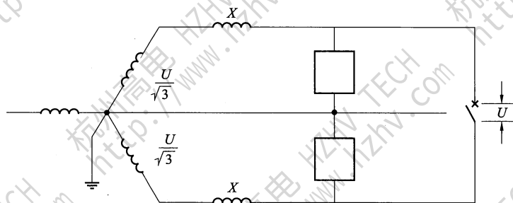
图 52 利用两个相差 120^\circ 的电压进行失步试验的试验回路
