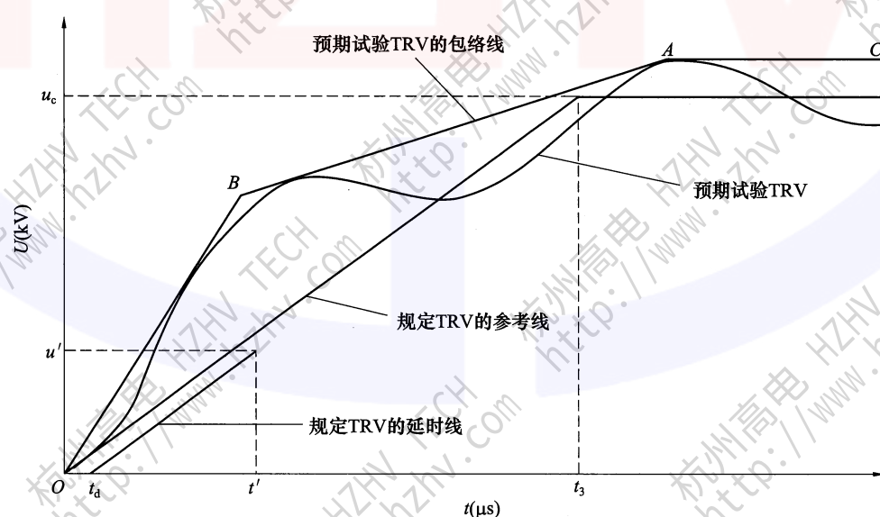
图 41 满足型式试验条件、用四参数包络线表示的预期试验的 TRV 示例： 具有两参数参考线的规定的 TRV 的情况
