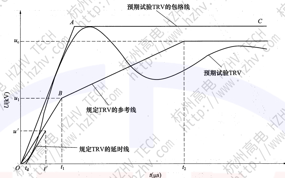
图 42 满足型式试验条件、用两参数包络线表示的预期试验的 TRV 示例： 具有四参数参考线的规定的 TRV 的情况
