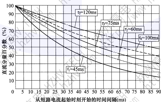
图9 对于标准时间常数 \tau_1 和特殊工况下的时间常数 \tau_2 、 \tau_3 、 \tau_4 及 \tau_5 ，直流分量的百分数与从短路起始时刻开始的时间间隔的关系曲线
