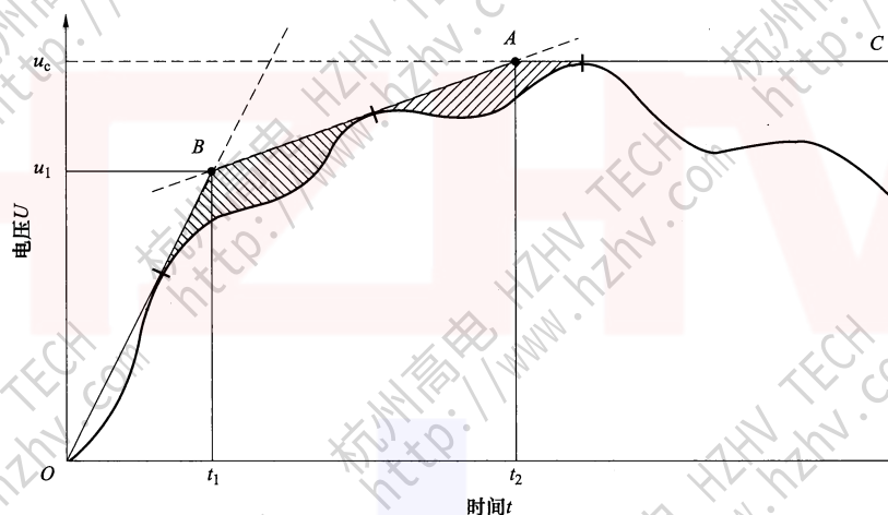
图 E.2 用四参数表示回路的预期瞬态恢复电压——E.2 中 b) 的情况
