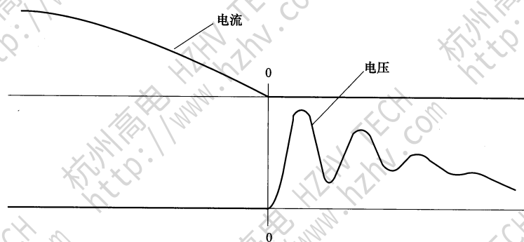
图 F.3 理想开断时的 TRV
