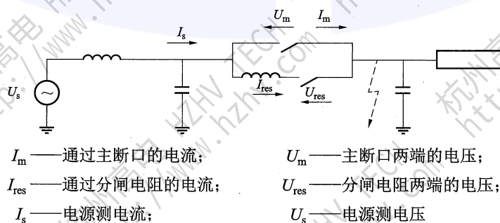
图 R.1 由带分闸电阻断路器开断的典型系统结构
