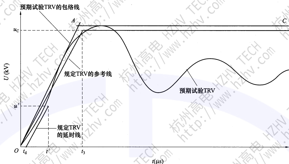
图 40 满足型式试验条件、用两参数包络线表示的预期试验的 TRV 示例： 具有两参数参考线规定的 TRV 的情况
