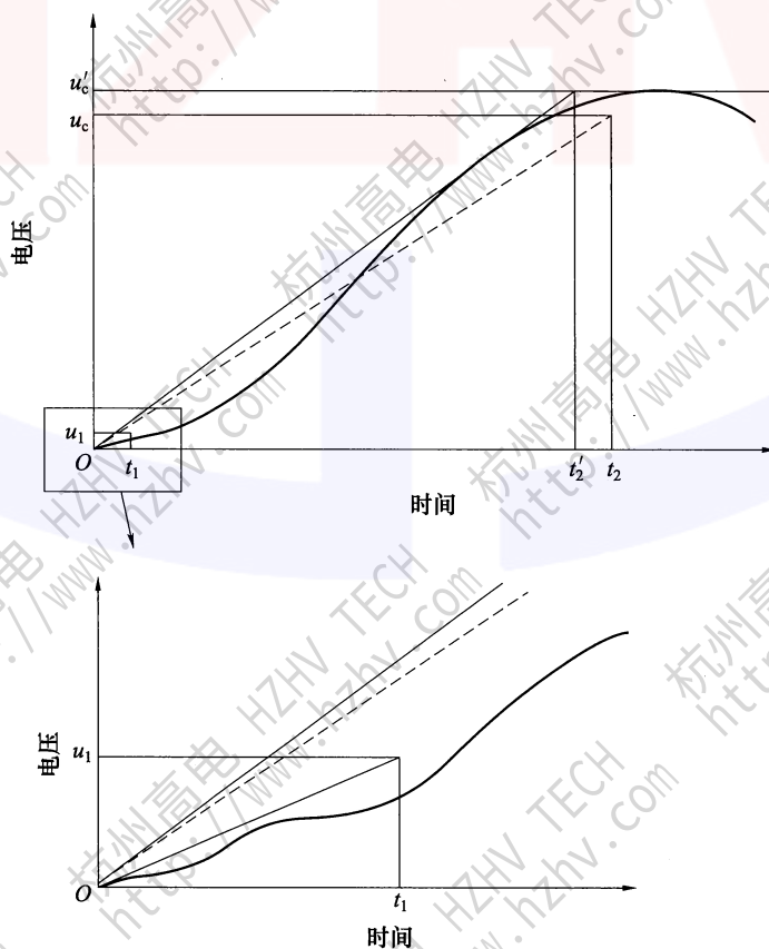
图 54 容性电流开断试验的恢复电压
