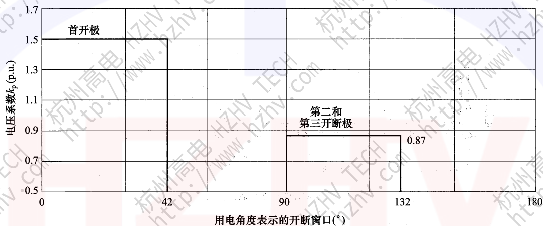
图 38 对于首开极系数为 1.5 的系统, 决定各极 TRV 的开断窗口和电压系数 k_p 的图形表示
