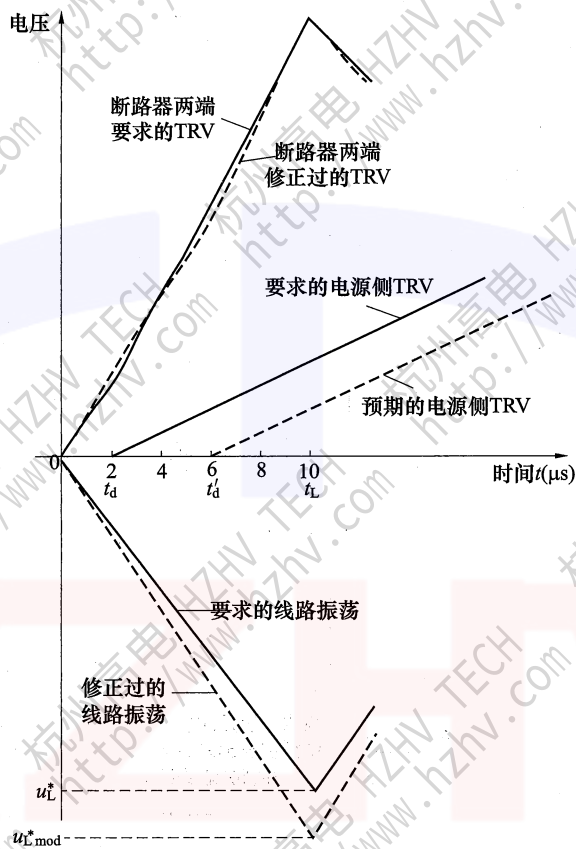
图 50 通过提高线路侧电压的幅值补偿电源侧延时的缺陷
