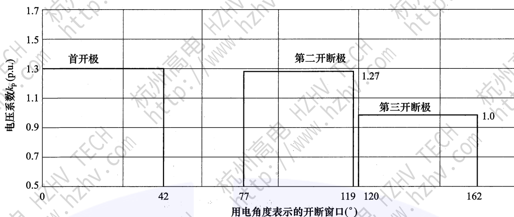
图 37 对于首开极系数为 1.3 的系统, 决定各极 TRV 的开断窗口和电压系数 k_p 的图形表示
