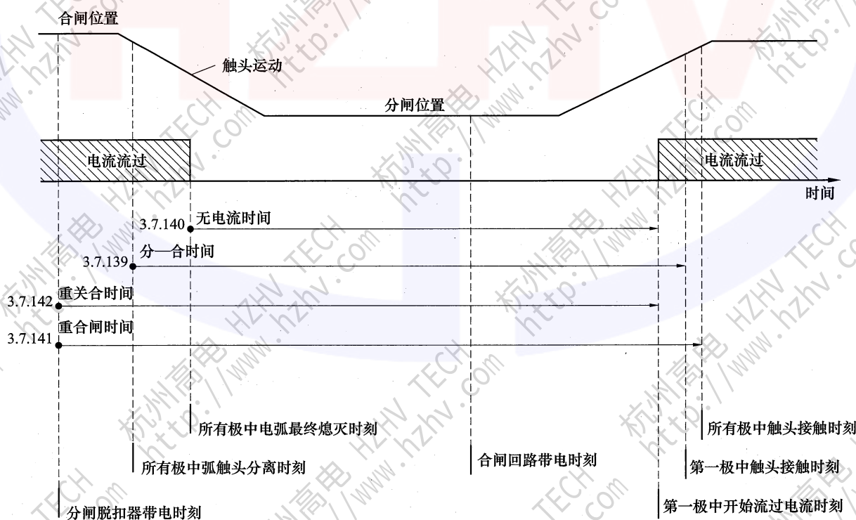
图 3 没有开合电阻的断路器的合—分循环
