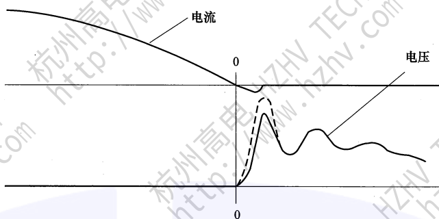
图 F.6 有弧后电流时的开断
