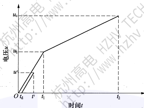
图 10 规定的四参数 TRV 及 T100、T60、 近区故障和失步条件的延时线的表示
