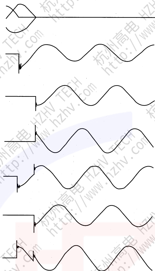
图 O.2 图 25 a) 所示表明三相开断过程中 对称电流、相对地和相间电压的波形示例
