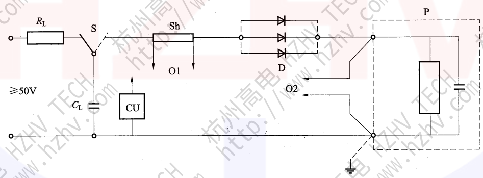
图 F.8 工频电流注入装置的操作顺序
