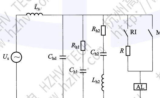
图 R.3 试验方式 T10、T30 和 OP2 的试验回路
