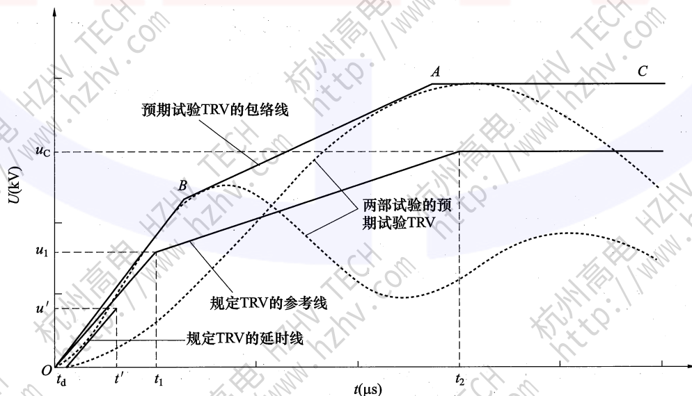
图 43 两部试验中两个预期的试验 TRV 波形及它们组合的包络线
