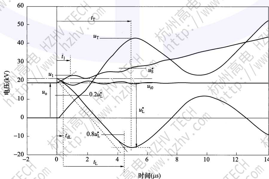
图 A.2 线路侧和电源侧 TRV 参数的典型图示——线路侧和电源侧均有延时；电源侧有 ITRV
