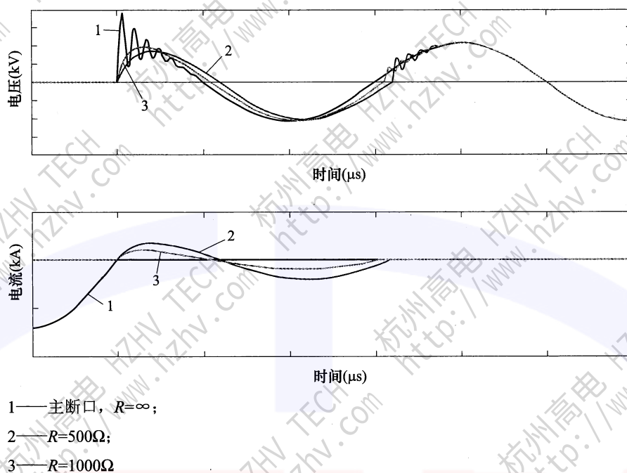
图 R.7 配有分闸电阻的断路器的电阻器断口上的 T10 (基于 U_r=1100\text{kV} 、 I_{sc}=50\text{kA} 和 f_r=50\text{Hz} ) 的典型恢复电压波形
