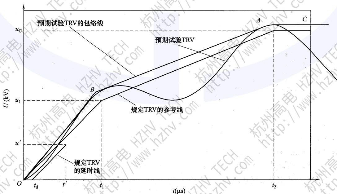
图 39 满足型式试验条件、用四参数包络线表示的预期试验的 TRV 示例: 具有四参数参考线规定的 TRV 的情况
