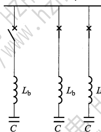
图 H.2 例 2 的回路图
