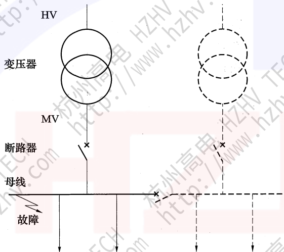
图 M.1 变压器限制故障的第一个事例 (也称为变压器馈电故障)
