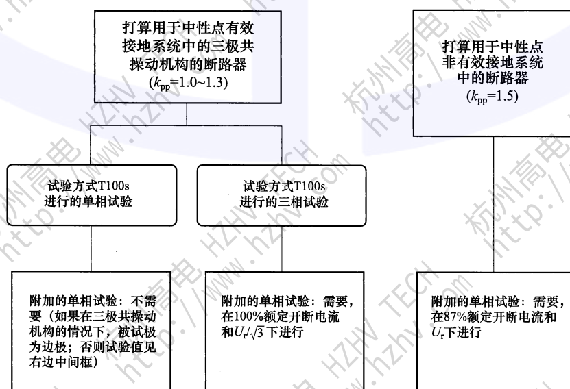
图 45 附加的单相试验的必要性和试验要求
